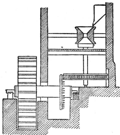
Водяная мельница. Реконструкция по Витрувию
